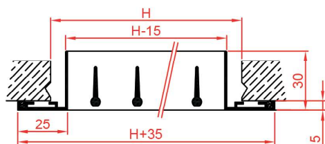
SDG avec registre de réglage (OBD)
