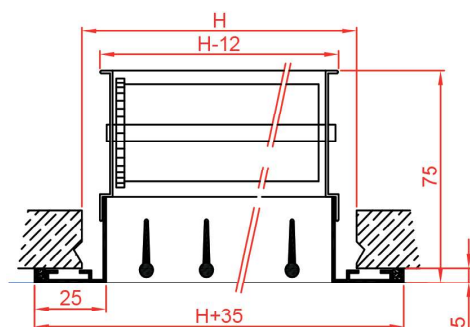
SDG avec registre de réglage (OBD)
